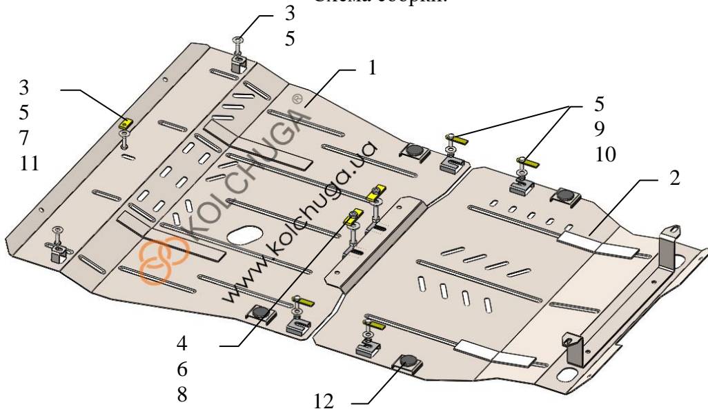
Схема сборки.
