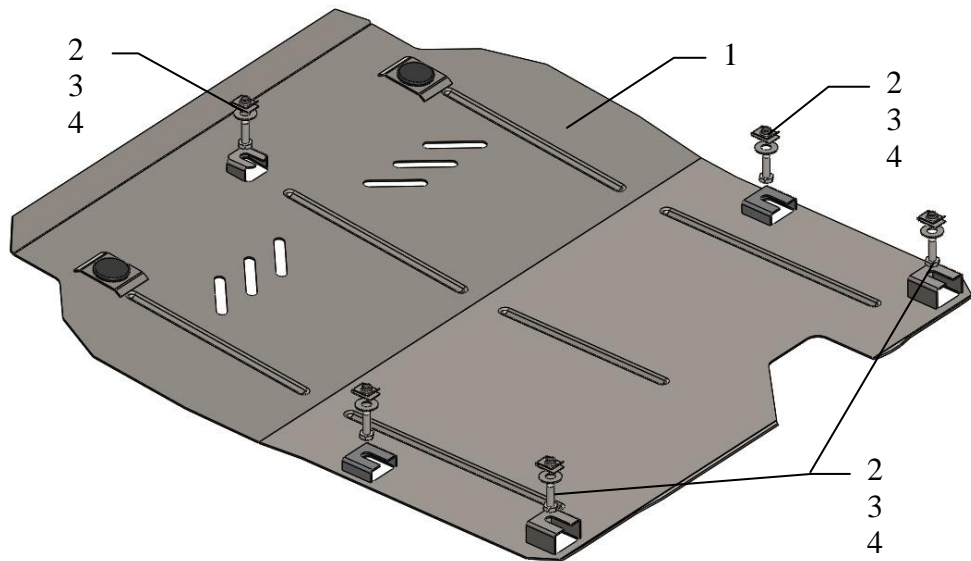
Схема сборки защиты картера и КПП.
