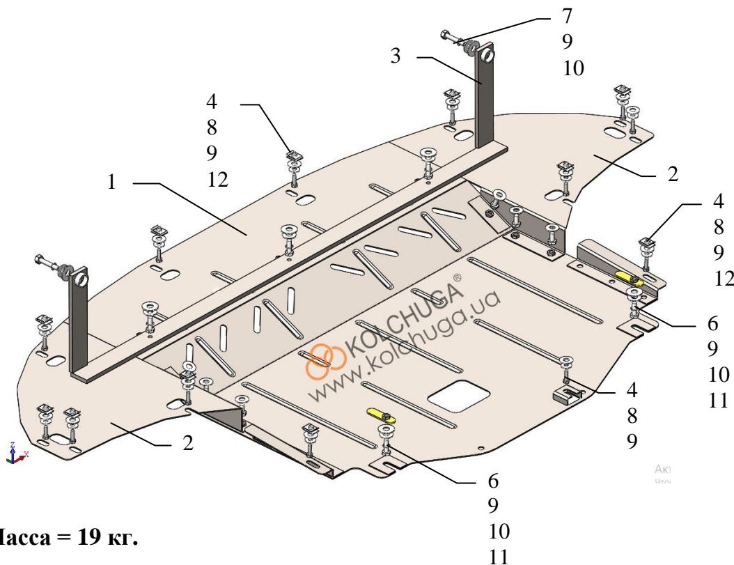
Схема сборки защиты радиатора, картера и КПП.
