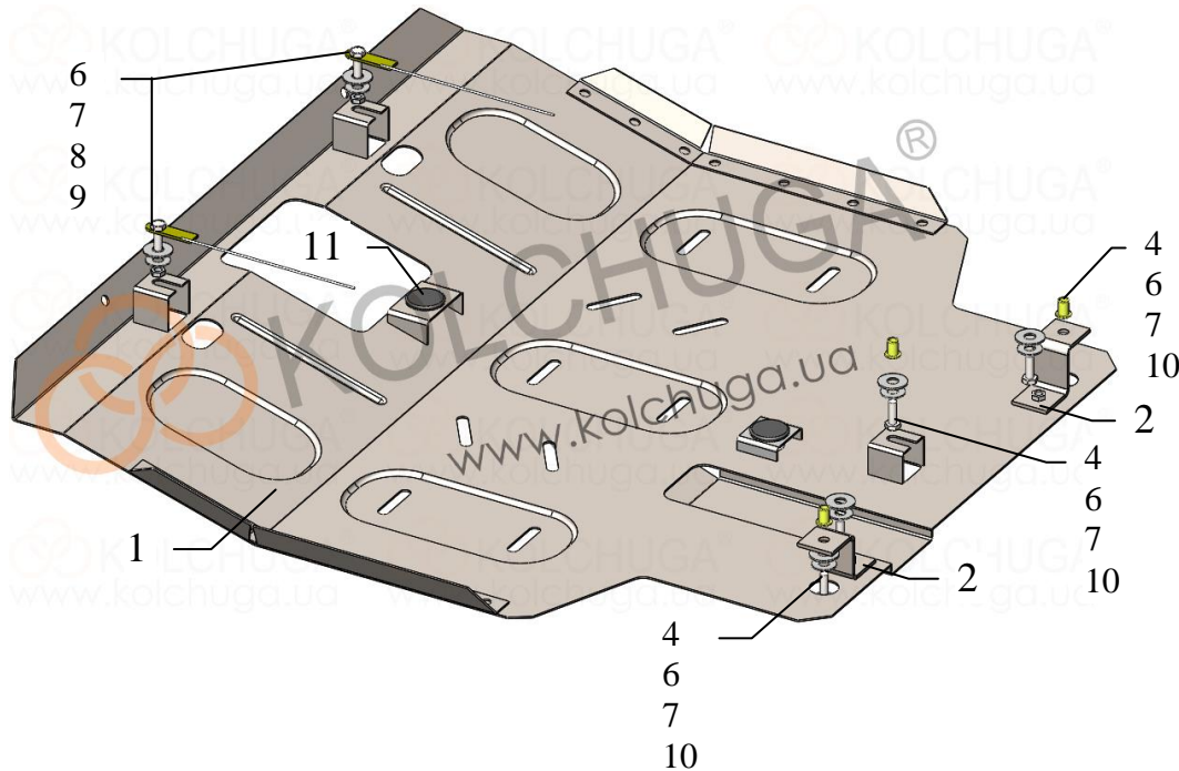
Схема сборки защиты радиатора, двигателя, КПП
